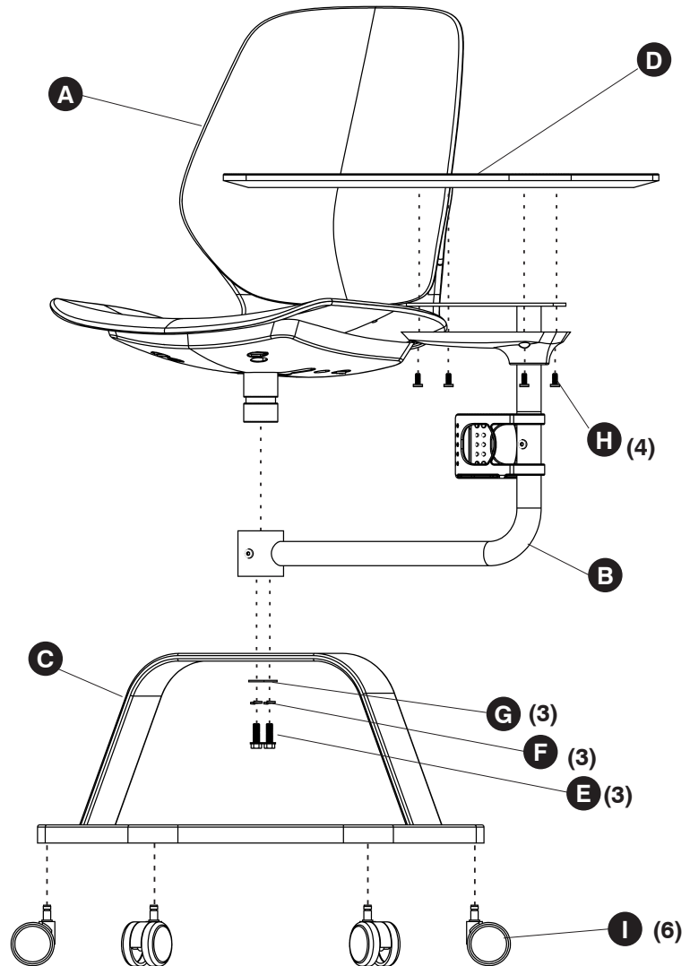
Lock Washer M8.5X15X2MM Rondelle de blocage M8.5X15X2MM Arandela de seguridad M8.5X15X2MM
